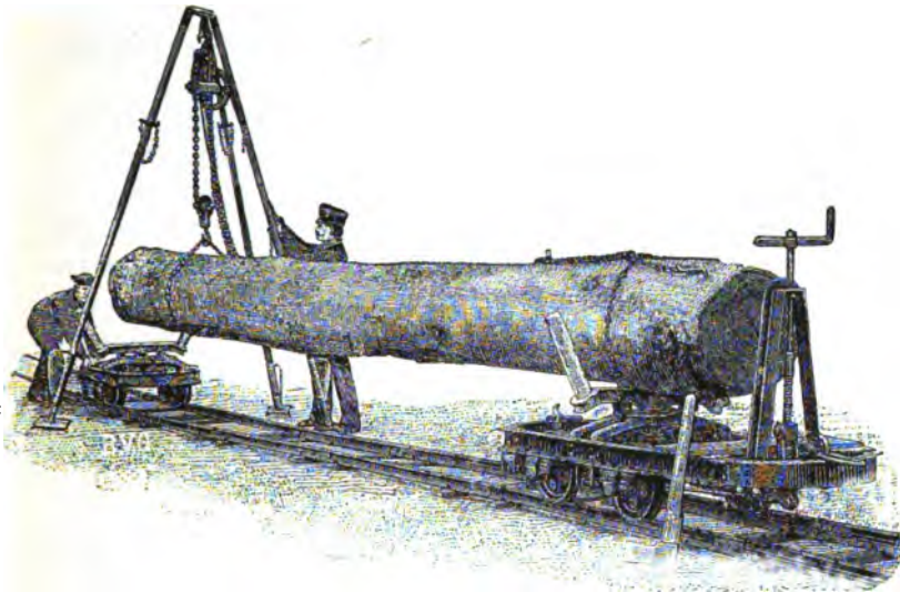
Fig. 216.—Simple crane.
